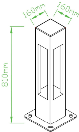
Outer Dimensions ————— Unit:mm
