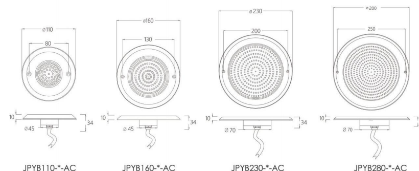
Outer Dimensions Unit:mm
